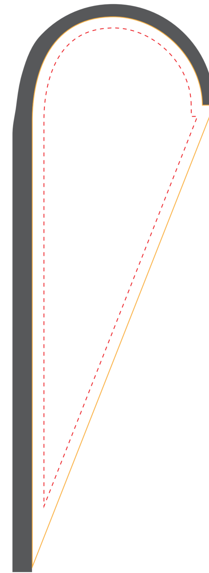
MOTION „D2“ GRÖSSE: 87 x 290 cm TUCHGRÖSSE: 87 x 245 cm
