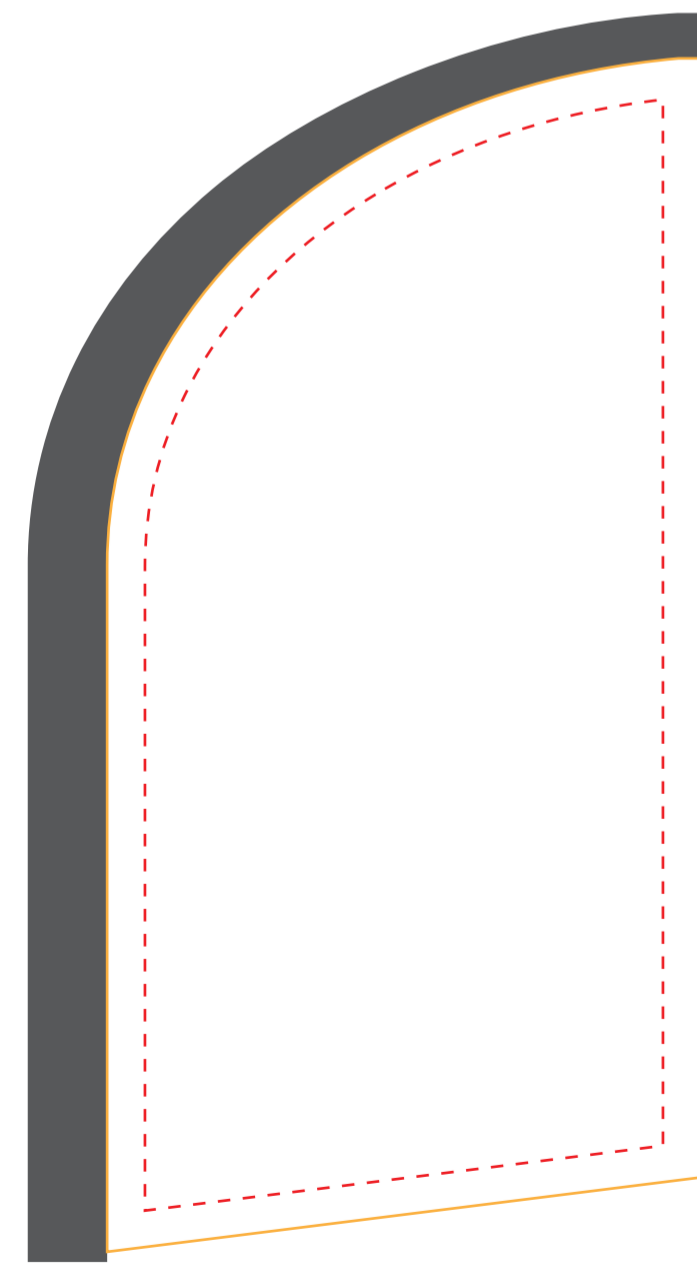
MOTION „C1“ GRÖSSE: 89 x 205 cm TUCHGRÖSSE: 89 x 165 cm
